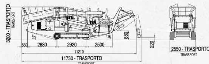
CONFIGURAZIONE DI TRASPORTO TRANSPORT CONFIGURATION
